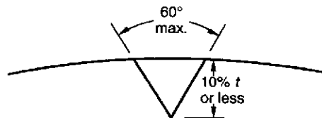
V10 NOTCH
