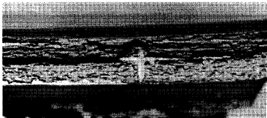
Figure 31b—Penetrators (ERW)
